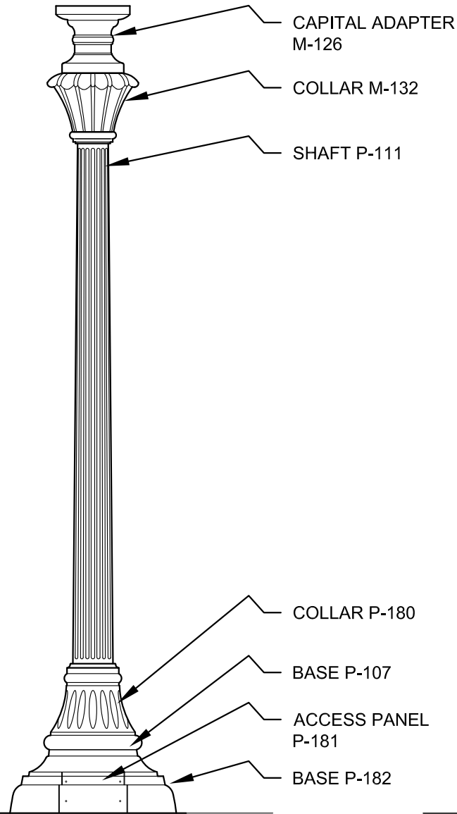
ELEVATION
